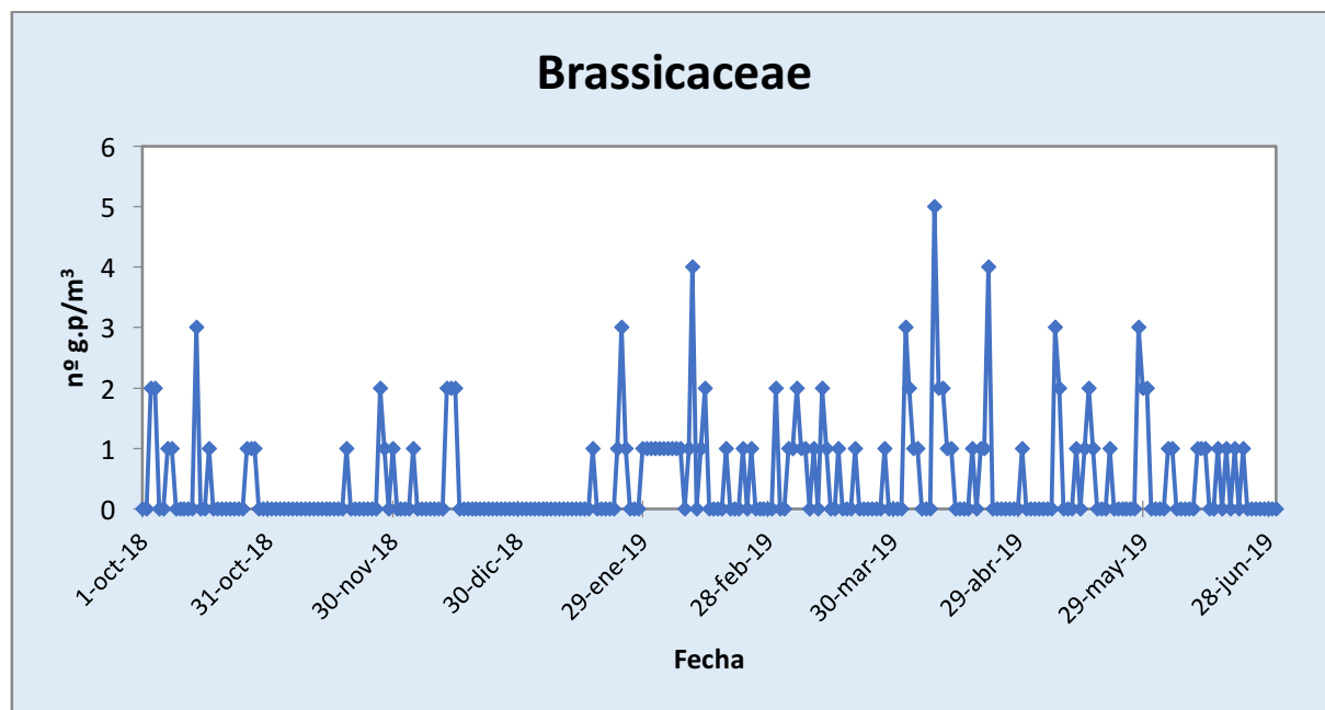
Figura 7. Comportamiento seguido por el polen de Brassicaceae en la atmósfera de Málaga-Centro durante el periodo octubre 2018-junio 2019.
