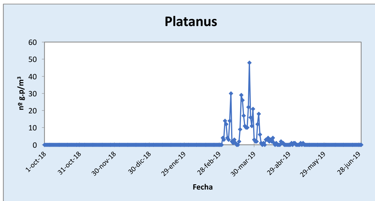
Figura 24. Comportamiento seguido por el polen de Platanus en la atmósfera de Málaga-Centro durante el periodo octubre 2018-junio 2019.
