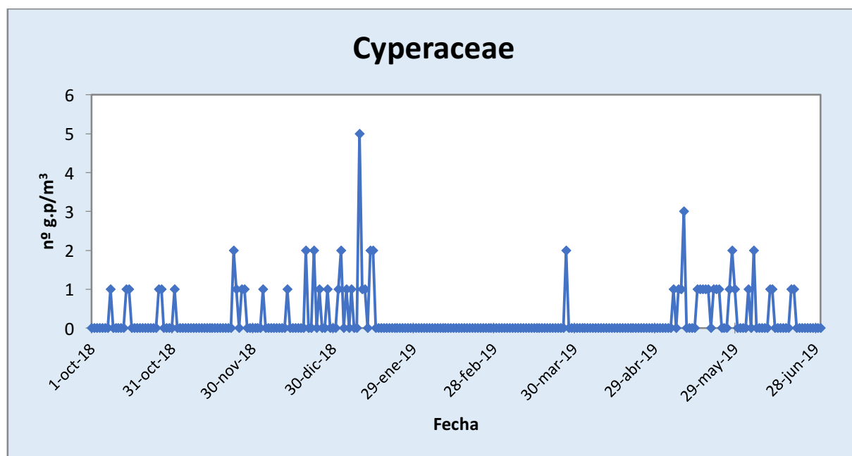
Figura 12. Comportamiento seguido por el polen de Cyperaceae en la atmósfera de Málaga-Centro durante el periodo octubre 2018-junio 2019.
