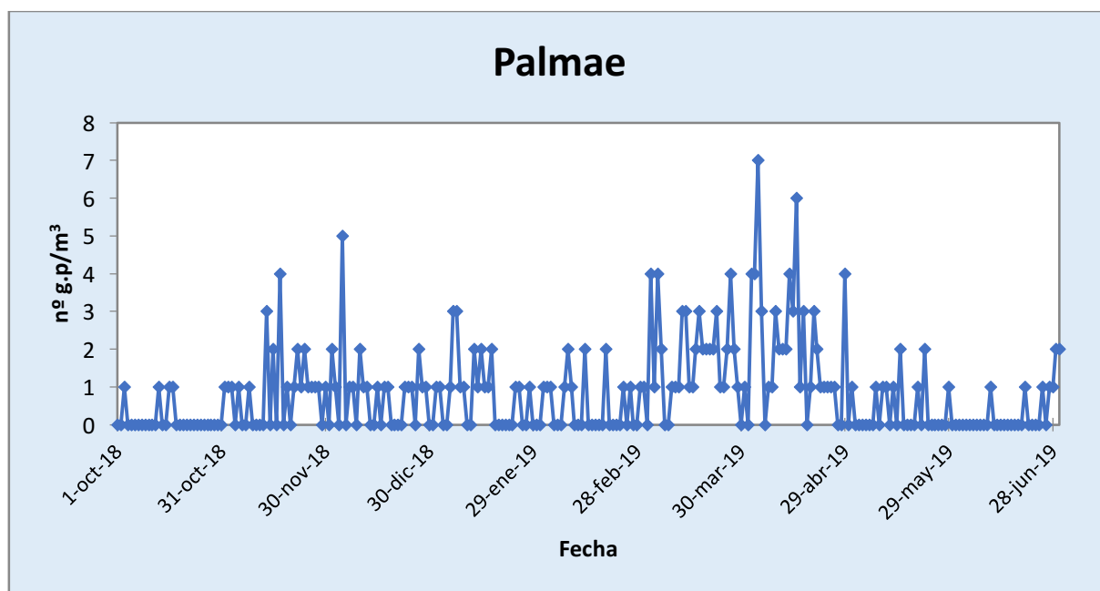
Figura 20. Comportamiento seguido por el polen de palmeras en la atmósfera de Málaga-Centro durante el periodo octubre 2018-junio 2019.
