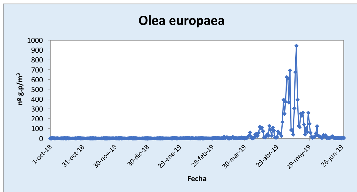
Figura 19. Comportamiento seguido por el polen de Olea europaea en la atmósfera de Málaga-Centro durante el periodo octubre 2018-junio 2019.
