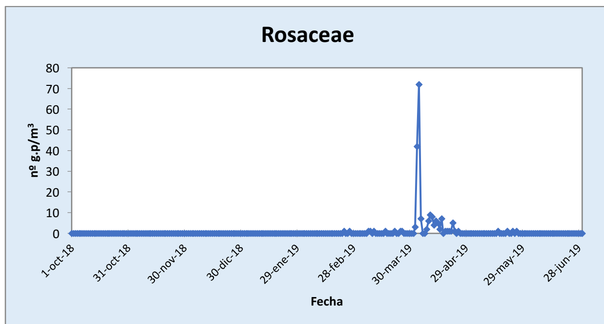
Figura 29. Comportamiento seguido por el polen de Rosaceae en la atmósfera de Málaga-Centro durante el periodo octubre 2018-junio 2019.
