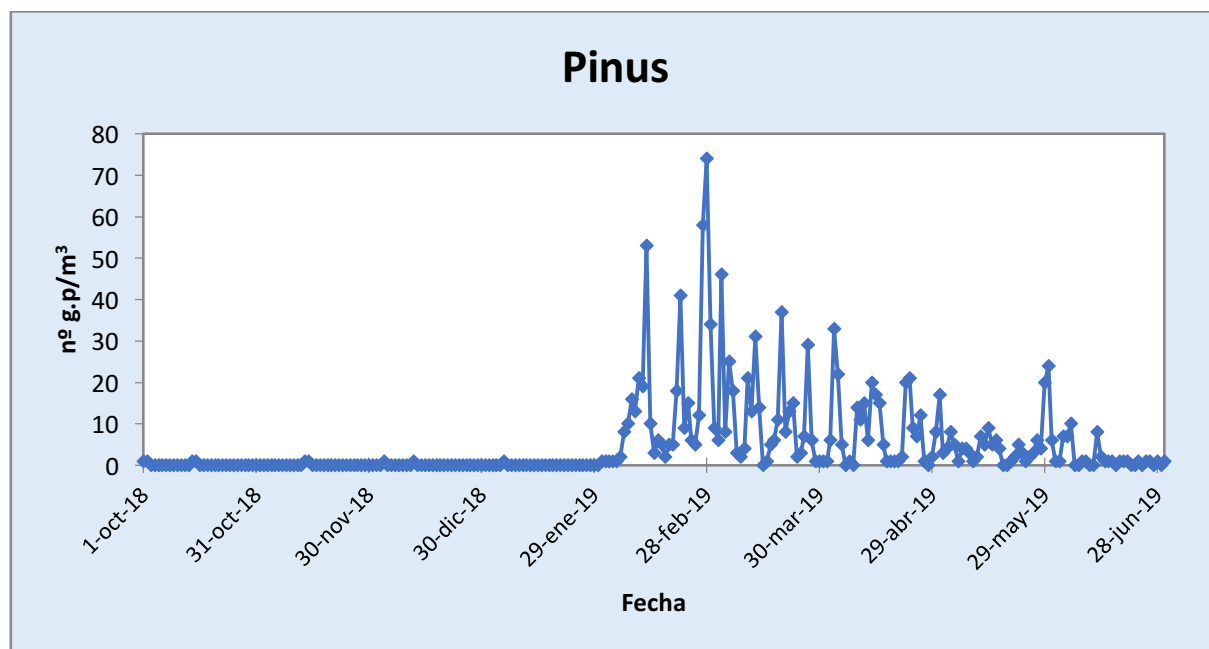
Figura 21. Comportamiento seguido por el polen de Pinus en la atmósfera de Málaga-Centro durante el periodo octubre 2018-junio 2019.
