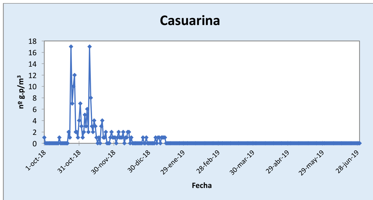
Figura 8. Comportamiento seguido por el polen de Casuarina en la atmósfera de Málaga-Centro durante el periodo octubre 2018-junio 2019.
