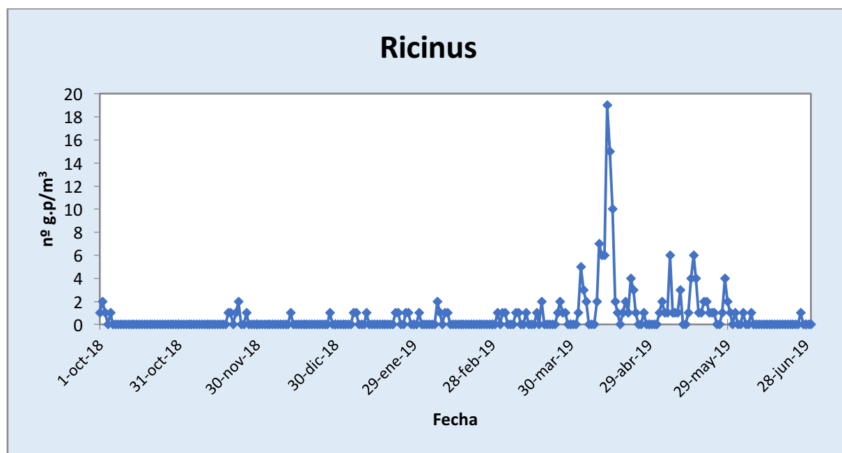
Figura28. Comportamiento seguido por el polen de Ricinus en la atmósfera de Málaga-Centro durante el periodo octubre 2018-junio 2019.
