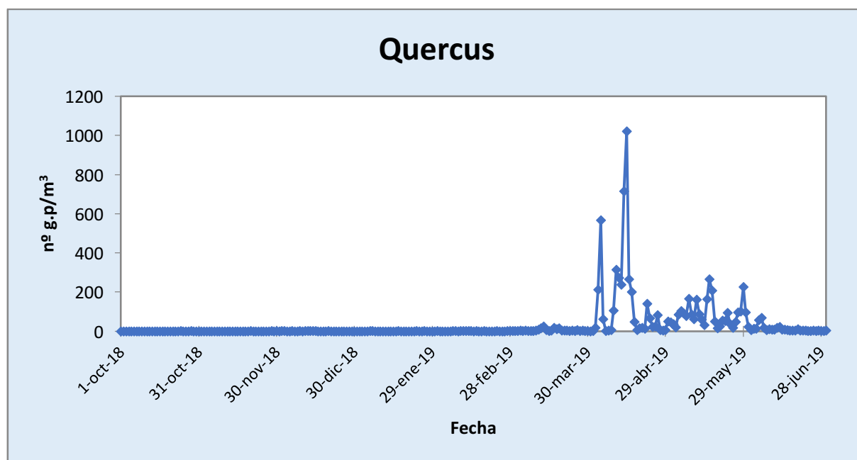
Figura 27. Comportamiento seguido por el polen de Quercus en la atmósfera de Málaga-Centro durante el periodo octubre 2018-junio 2019.
