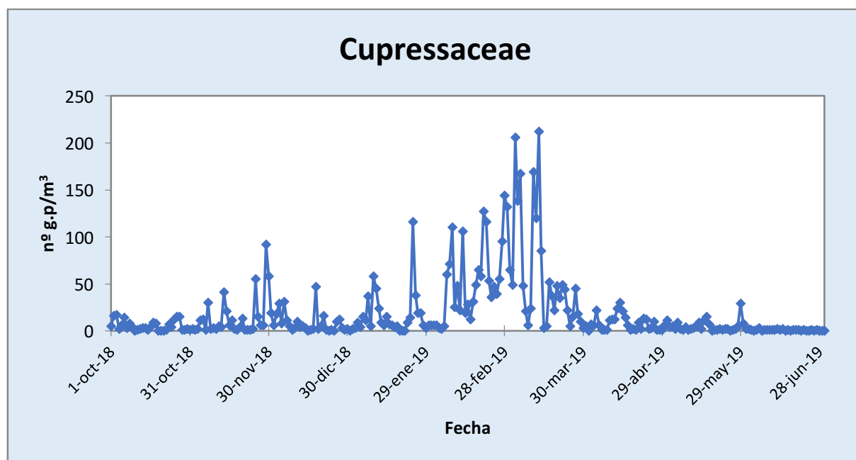
Figura 11. Comportamiento seguido por el polen de Cupressaceae en la atmósfera de Málaga-Centro durante el periodo octubre 2018-junio 2019.
