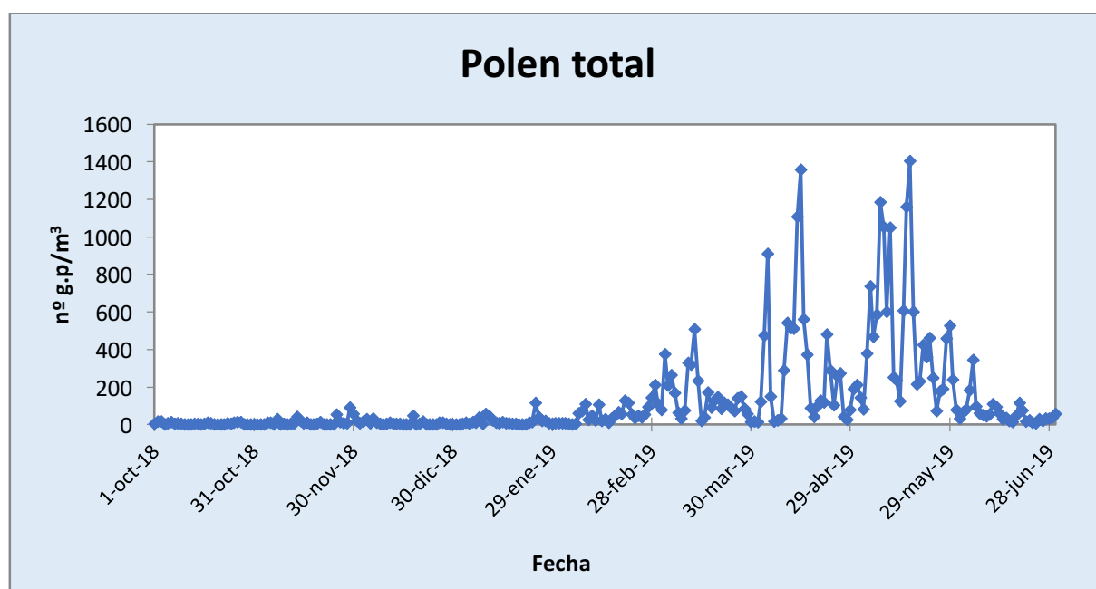
Figura 3. Comportamiento seguido por el polen total en la atmósfera de Málaga-Centro durante el periodo octubre 2018-junio 2019.
