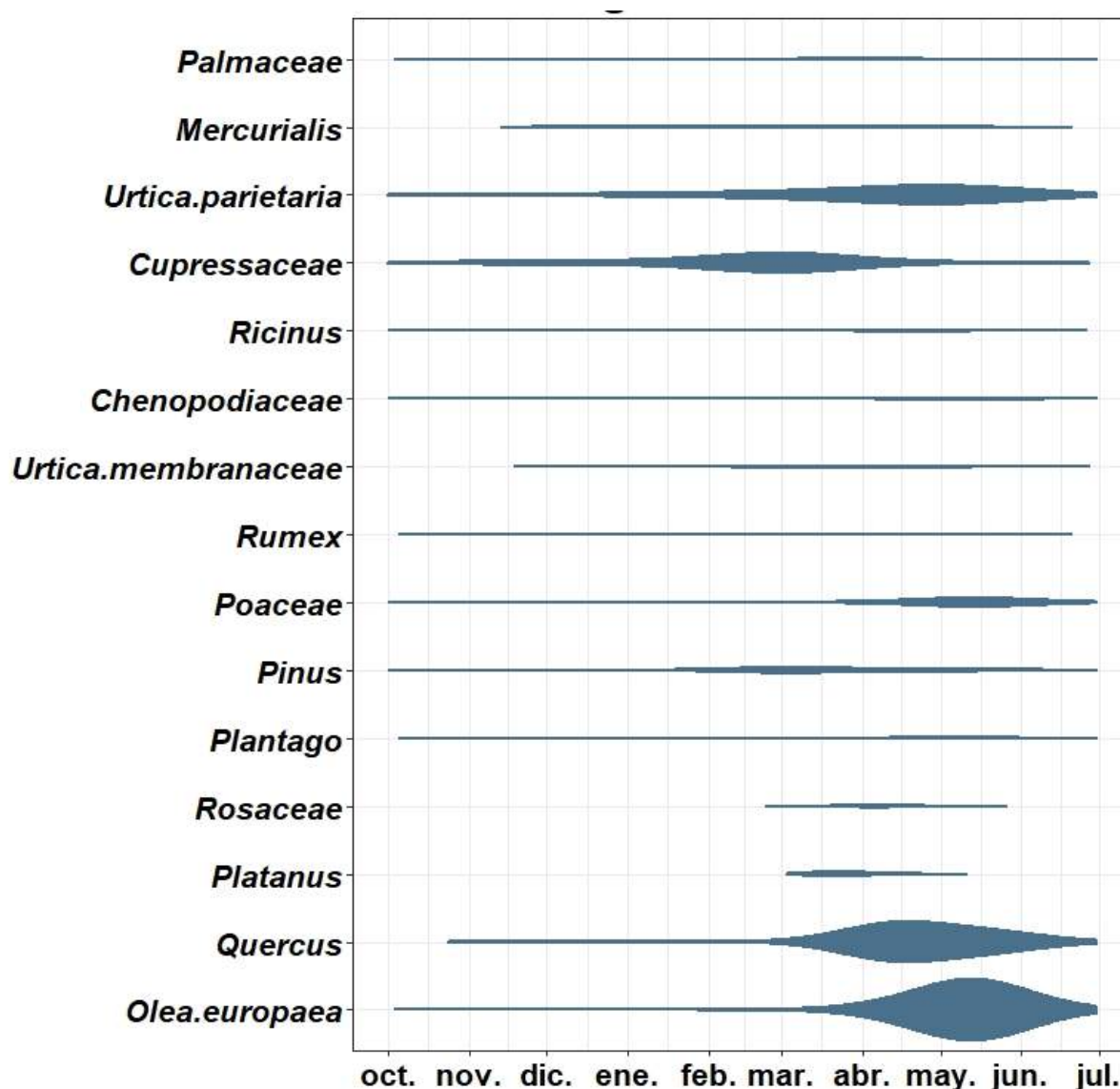
Figura 33. Calendario polínico observado en la atmósfera de la estación Málaga-Centro durante el periodo octubre 2018-junio 2019.
