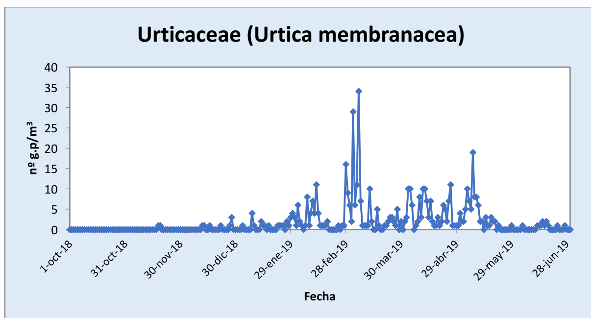
Figura 32. Comportamiento seguido por el polen de Urtica membranacea en la atmósfera de Málaga-Centro durante el periodo octubre 2018-junio 2019.
